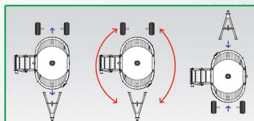
GRÁFICO DEMOSTRATIVO DE LA FORMA Y CAMBIO DE POSICIÓN DE LANZA Y EJE.
